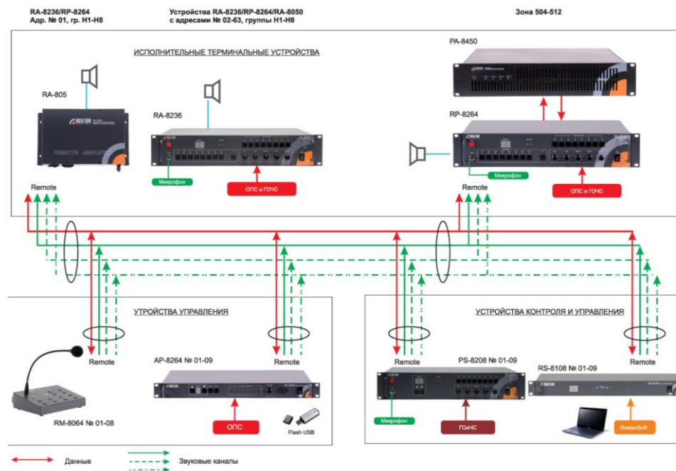
Рисунок 1. Структурная схема соединения компонентов ROXTON 8000
